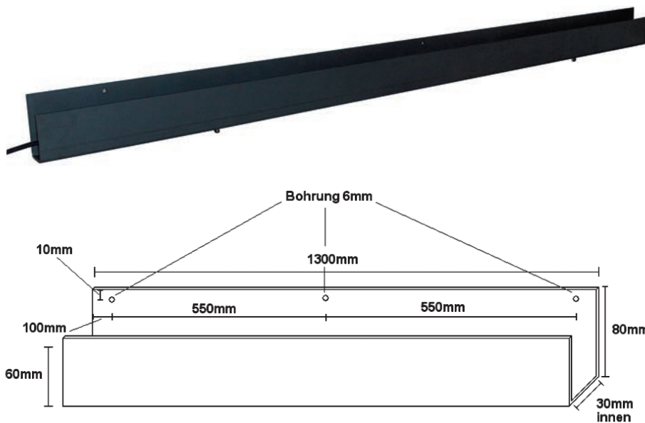
Stahlprofil S235 3mm
